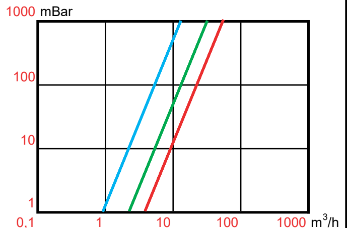
Diagramma log. perdite di carico / portata Load losses / flow rate log.graph
