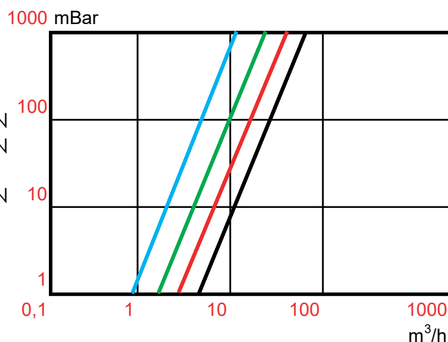
Diagramma log. perdite di carico / portata Load losses / flow rate log.graph
