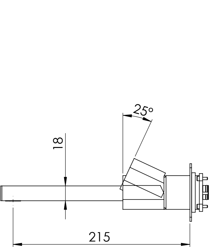
CONNESSIONE DEVIATORE D522AWBAB CONNECTION DIVERTER D522AWBAB
