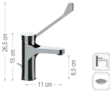
LL10 Miscelatore monocomando lavabo, con scarico. Single-lever basin mixer, with pop-up waste.
