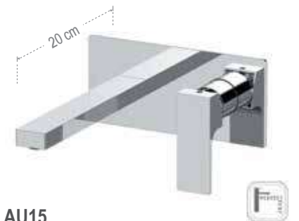
AU15 Miscelatore monocomando a incasso per lavabo, in ottone, lunghezza bocca 20 cm. Single-lever built-in basin mixer, in brass, spout length 20 cm.
