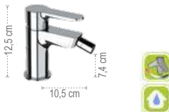
WE22LT6 Miscelatore monocomando per bidet, senza scarico e senza foro posteriore sul corpo. Single-lever bidet mixer, without waste and without rear body hole.
