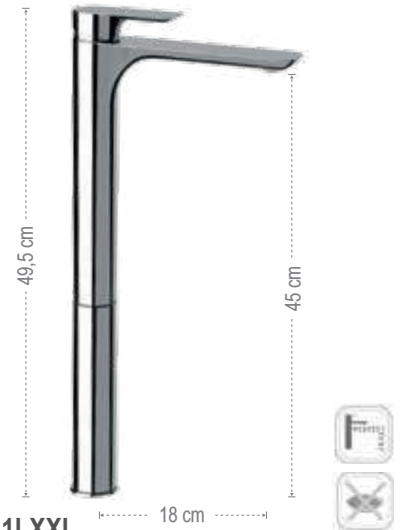
I11LXXL Miscelatore monocomando lavabo alto XXL, senza scarico. XXL high single-lever basin mixer, without waste.
