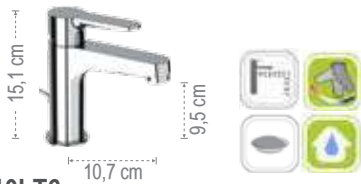
WE10LT6 Miscelatore monocomando lavabo, con scarico. Single-lever basin mixer, with pop-up waste.
