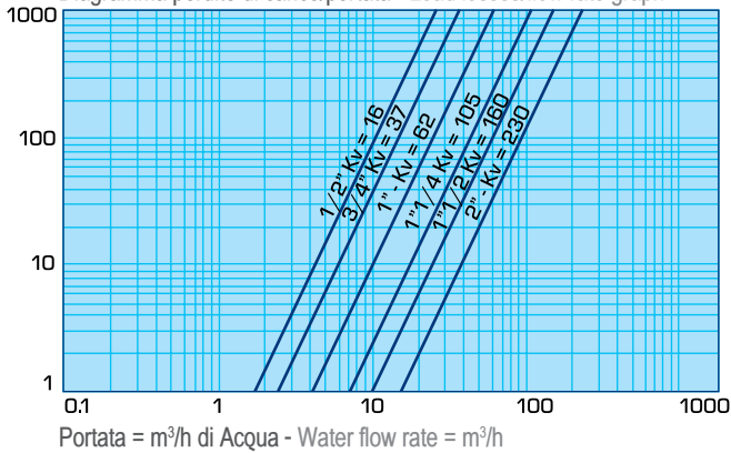
Diagramma perdite di carico/portata - Load losses/flow rate graph
