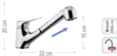
G474 Miscelatore monocomando per lavello, con doccia estraibile a getto variabile. Single-lever one-hole sink mixer, with pull-out spray jet shower, 2 functions.
