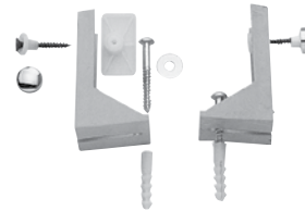
Coppia zanche in plastica antiurto a L con viti, per fissaggio laterale W.C. e bidet. Couple wall brackets in plastic, shock-resistant, L shaped, with screws, for side WC and bidet fixing.
