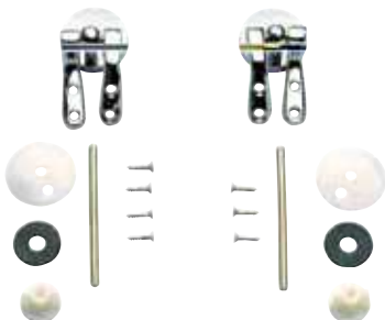
Coppia cerniere per fissaggio sedili W.C. in legno, con 8 viti in ottone. Couple hinges for fixing W.C. seats, with 8 screws.
