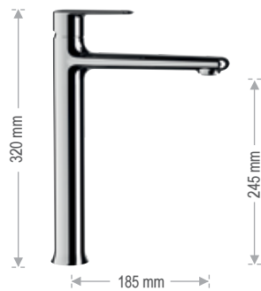
V 10 L Miscelatore monocomando lavabo. Single-lever basin mixer.
