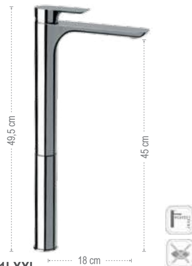
I11LXXL Miscelatore monocomando lavabo alto XXL, senza scarico. XXL high single-lever basin mixer, without waste.
